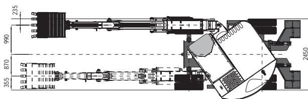
Abb. 1: Spurdeckendes Baggern
